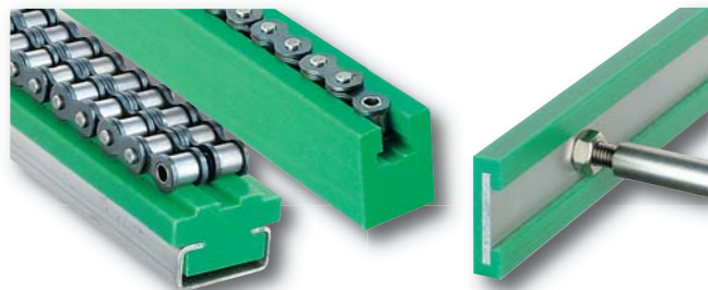
Profils de glissement et guides chaînes.
